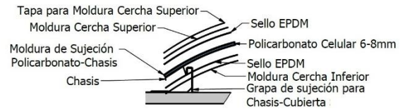
Fig. 1.2 Componentes Generales del Sistema Arco Cañón THERMABLOK
